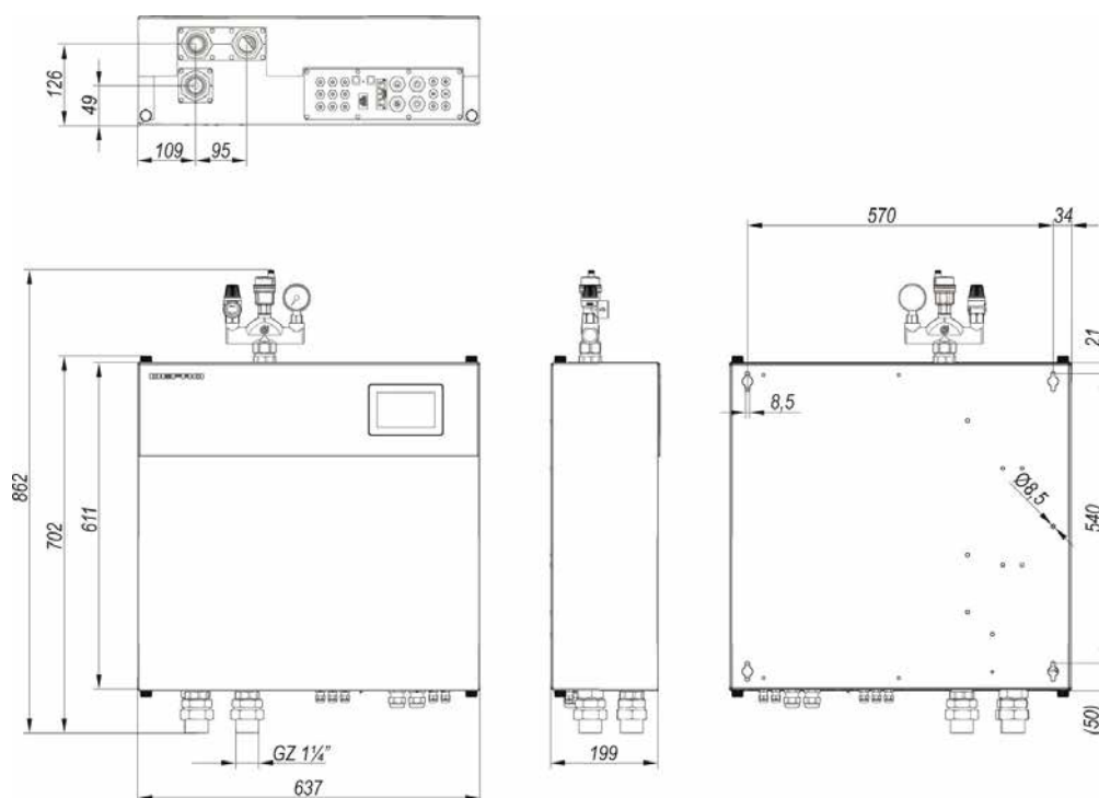
Rozměry hydromodulu DFi tepelného čerpadla DHPi MONOTEC 16 a DHPi MONOTEC 20
