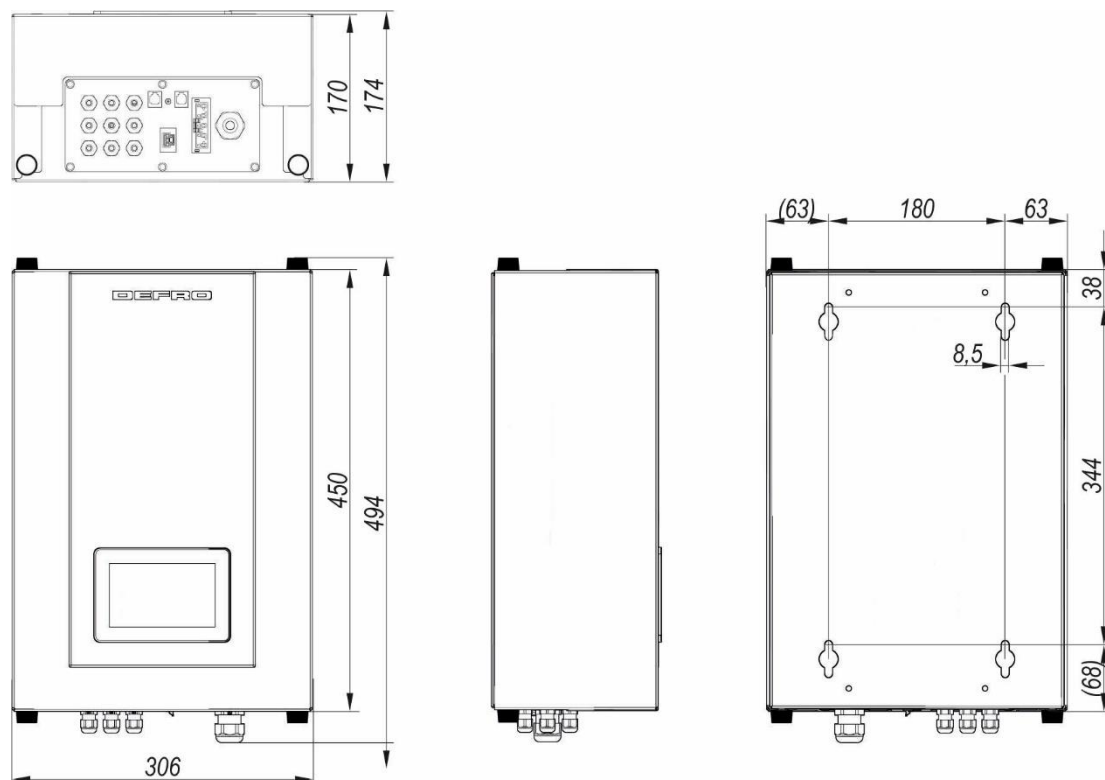
Rozměry instalační skříňky DSi tepelného čerpadla DHPi MONOTEC
