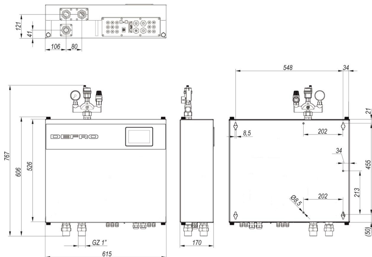
Rozměry hydromodulu DFi tepelného čerpadla DHPi MONOTEC 8 a DHPi MONOTEC 12
